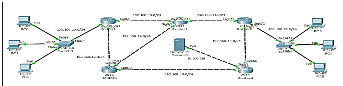
Gambar 1. Skema jaringan
